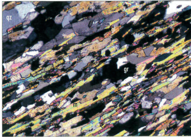
Microscopie de pétrographie, lumière polarisée et analysée, grossissement de 10 fois. La roche est un schiste bleu à glaucophane et à grenat, fréquent dans toute l'unité du Diahot, jusqu'au Mont Panié. Les minéraux colorés en jaune (teintes de polarisation vives) sont des baguettes d'une amphibole bleue (glaucophane) caractéristique de transformations métamorphiques à haute pression. Les autres minéraux vivement colorés sont des paillettes de micas. Ces deux minéraux montrent une orientation préférentielle qui détermine une organisation en feuillets. Des cristaux noirs de grenats ponctuent cette roche.
