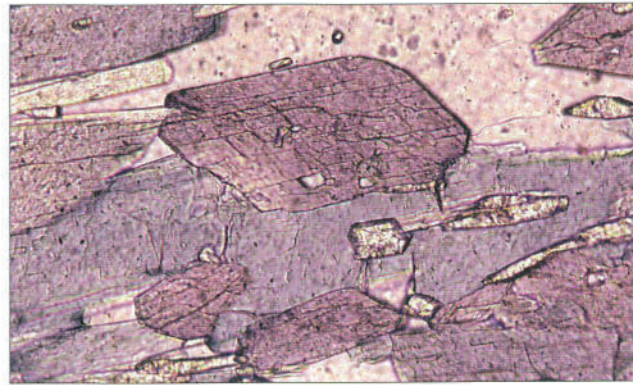
Microscopie de pétrographie, lumière polarisée, grossissement de 10 fois. Les schistes bleus du bassin du Diahot n'ont pas pris cette couleur par hasard. Ils sont chargés de petites baguettes d'une amphibole dont la couleur, en lumière polarisée, varie du bleu au violet. Les sections transversales, perpendiculaires à l'axe d'allongement des baguettes, font apparaître deux familles de microfissures (plans de clivage), disposées selon un angle de 120°.
