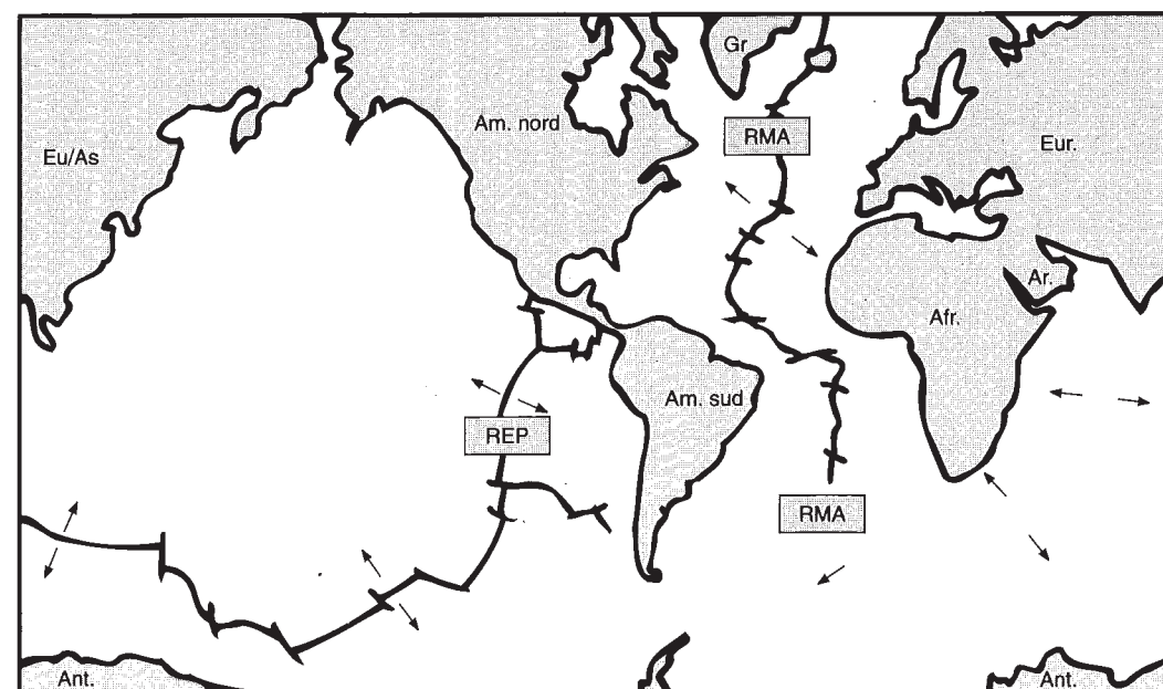
REP : ride est-Pacifique RMA : ride médio-atlantique ← → divergence entre deux plaques de part et d'autre d'une dorsale
