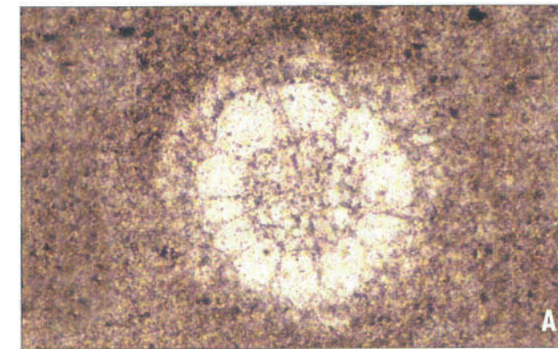
Microscopie de pétrographie, lumière polarisée, grossissement de 100 fois.
