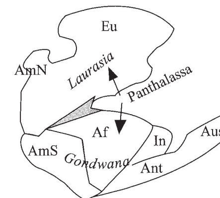
La position des continents à la fin du Primaire (-245 Ma)
