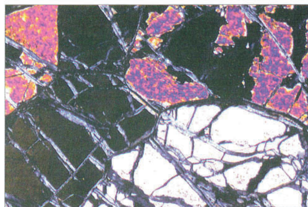
Microscopie de pétrographie, lumière polarisée et analysée, grossissement de 10 fois. Péridotite (dunite) serpentinisée. Les 4 ou 5 cristaux d'olivine sont parcourus par un réseau de micro-filons de serpentine (grise) qui semble les découper en un grand nombre de petits cristaux.
