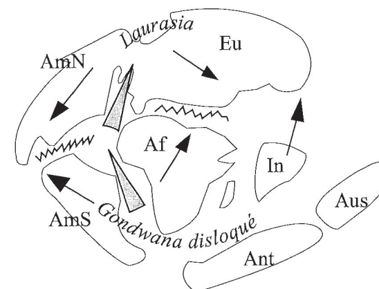
La position des continents à la fin du Secondaire (-65 Ma)
