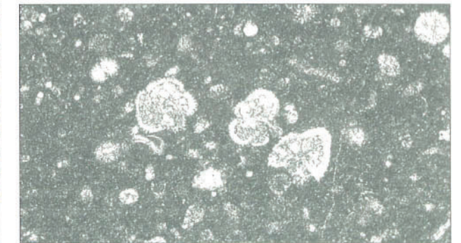
Microscopie de pétrographie, lumière polarisée, grossissement de 50 fois.
