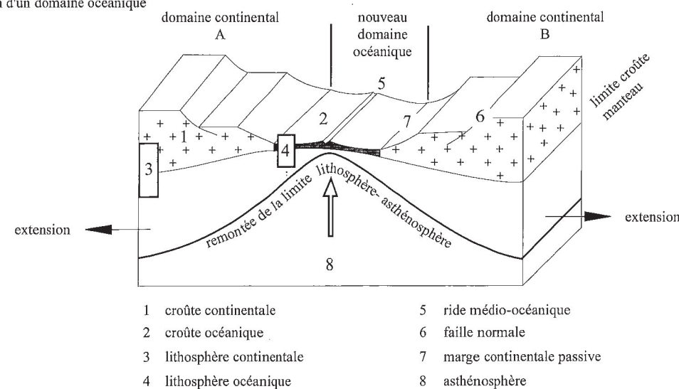
Structures accompagnant la fragmentation de la lithosphère quand deux masses continentales se séparent
