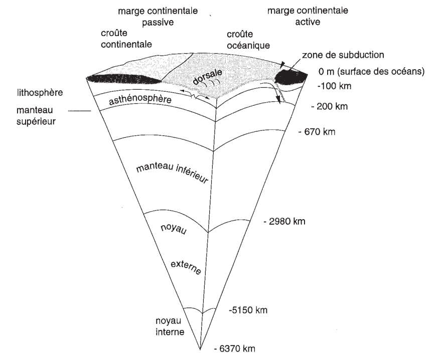
La structure du globe terrestre:
