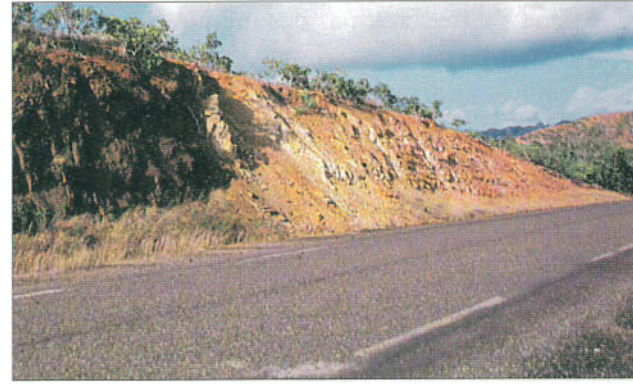
RPN1, entre Koumac et Poum, Malabou-beach, nord de la Grande Terre. Dans les schistes du bassin de l'unité du Diahot (zone claire du talus) sont intercalés des basaltes métamorphisés (zone sombre du talus). Ces deux matériaux réagissent différemment aux contraintes mécaniques développées lors des événements tectoniques. Les schistes présentent un débit caractéristique en feuillets alors que les basaltes sont simplement fracturés.
