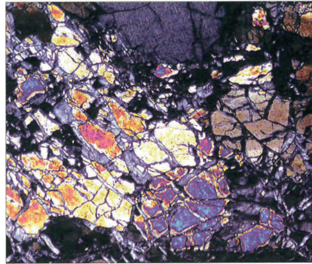
Microscope de pétrographie, lumière polarisée et analysée, grossissement de 20 fois. La serpentinisation des péridotites a été un processus préalable nécessaire à la genèse des minerais de nickel. Les grains d'olivine, aux teintes de polarisation vives, sont découpés par un réseau de filaments de serpentines (grises). Le gros cristal de pyroxène, presque noir, est exempt de serpentinisation.
