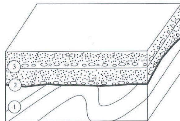
1 : dépôt, érosion et plissement de roches sédimentaires anciennes 2 : surface d'érosion 3 : dépôt en discordance de terrains postérieurs au plissement.
