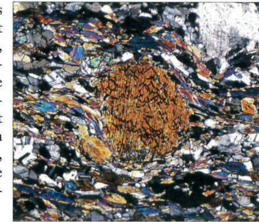
Microscopie de pétrographie, lumière polarisée et analysée, grossissement de 10 fois. Le jade de l'île Ouvéa est une roche métamorphique. Le gros cristal (au centre) est une relique de pyroxène magmatique (deux clivages orthogonaux et un troisième oblique, plus fin) rappelant que le jade dérive d'un gabbro. Les petits cristaux colorés, formés dans les conditions du métamorphisme, sont des amphiboles (néphrite) qui donnent sa couleur verte à la roche. Une organisation en feuillets montre que ces matériaux ont subi quelques contraintes mécaniques au cours de leur histoire métamorphique.
