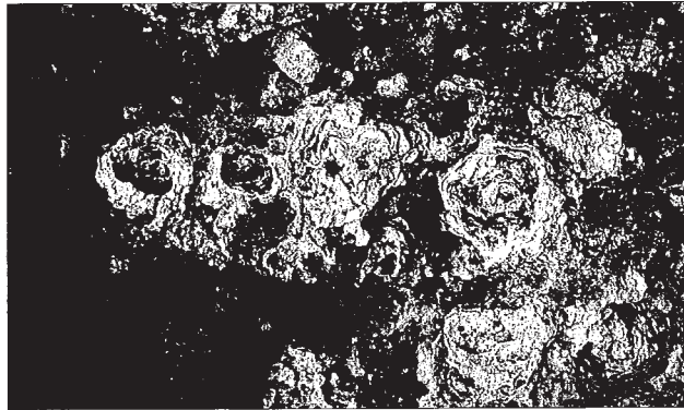
Calcaires à rhodolithes L'essentiel des îles Loyauté est constitué de calcaires associant des algues rouges et des grands foraminifères : les rhodolithes. Ces fossiles, accumulés sur une grande épaisseur, ont commencé à se développer il y a une quinzaine de millions d'années à une époque où la température des eaux de surface, plus basse qu'actuellement de 5 degrés, interdisait l'installation des coraux.
