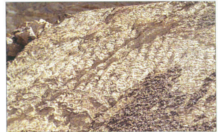
RP 2, route du Mont Dore, versant ouest. La surface de certains bancs de grès du Crétacé supérieur est parcourue de vaguelettes ou "ripple-marks". Ces figures rappellent celles laissées sur le sable des plages par des remous (courants, vagues). Cette observation suggère que, lors de leur dépôt il y a 80 millions d'années, ces grès étaient soumis à des conditions analogues. Le littoral ne devait pas être loin.
