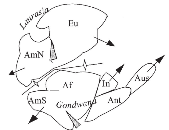
La position des continents au Jurassique (entre -180 et -160 Ma)
