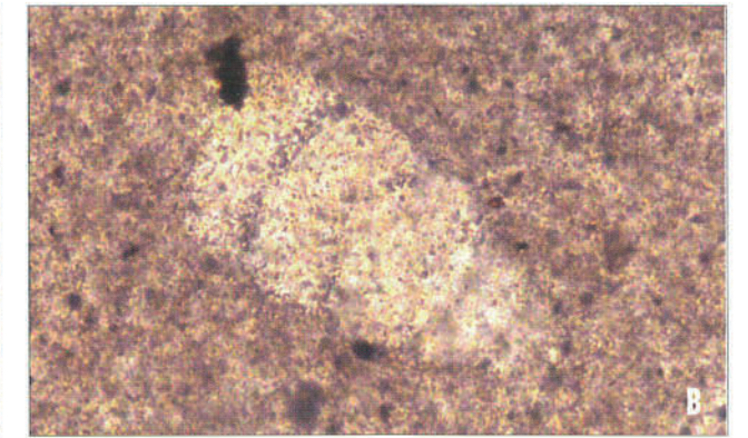
Nouméa, Ouen-Toro, entre la piscine et la côte blanche. Les roches plissées sont ici des phtanites, roches sédimentaires riches en silice, d'origine biologique et déposées en milieu marin profond. Leur dépôt est contemporain de celui des calcaires de Nouville, c'est-à-dire vieux de 60 à 45 millions d'années.
