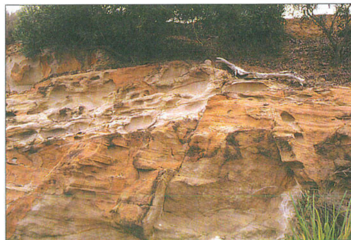
Nouméa, RP 14, face à l'aérodrome de Magenta. Les grès déposés au Crétacé supérieur, riches en débris de feldspath, prennent ici une teinte rouille en raison de l'oxydation de nombreux grains de pyrite. Celle-ci est présente dans les niveaux riches en matière organique. La stratification est quasiment horizontale, seulement interrompue par des failles. Quelques niveaux plus grossiers apparaissent en relief.
